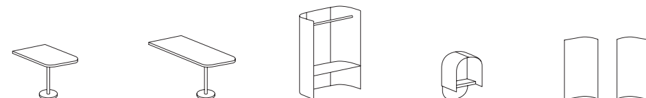
SR/WR/DLS/S 100 x 85 x 73 SR/WR/DHS/S 100 x 85 x 73 SR/WR/DHSR/S 167 x 85 x 73 SR/WR/TLS/S 167 x 85 x 73 SR/WR/THS/S 167 x 85 x 73 SR/WR/THSR/S 167 x 85 x 73 SR/CR 134 x 66 x 191 x 43 SR/PB 67 x 49 x 101 SR/CLP 67 x 34 x 136
