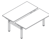
BOD576 1600 / 1490 / 700-1200 102,1 kg
