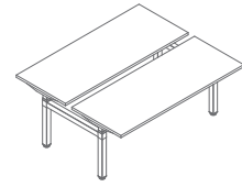
BOD578 1800 / 1490 / 700-1200 104,1 kg
